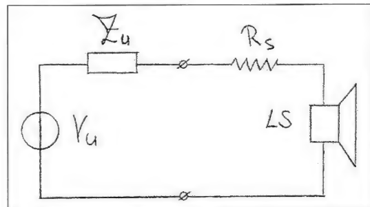
fig.21 Spanningversterker bestaat uit een ideale spanningsbron ( V_u ) en de uitgangsimpedantie ( Z_u ). De luidspreker bestaat uit een ideale luidspreker en een serie weerstand ( R_s ).
